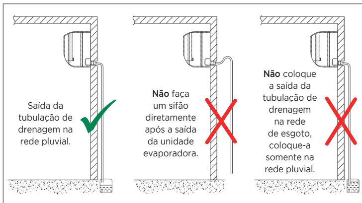
FIG. 7 - EXEMPLOS DE SITUAÇÕES DE DRENAGEM
