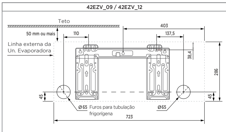
FIG. 11 - SUPORTES DE MONTAGEM
