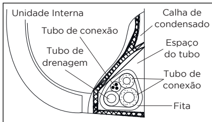
FIG. 8 - TUBO DE CONEXÕES
